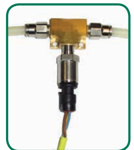
Druckluftaufnehmer
